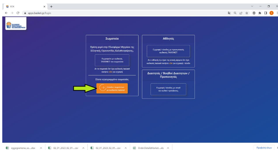
Εικόνα 1: Αυθεντικοποίηση σωματίου
