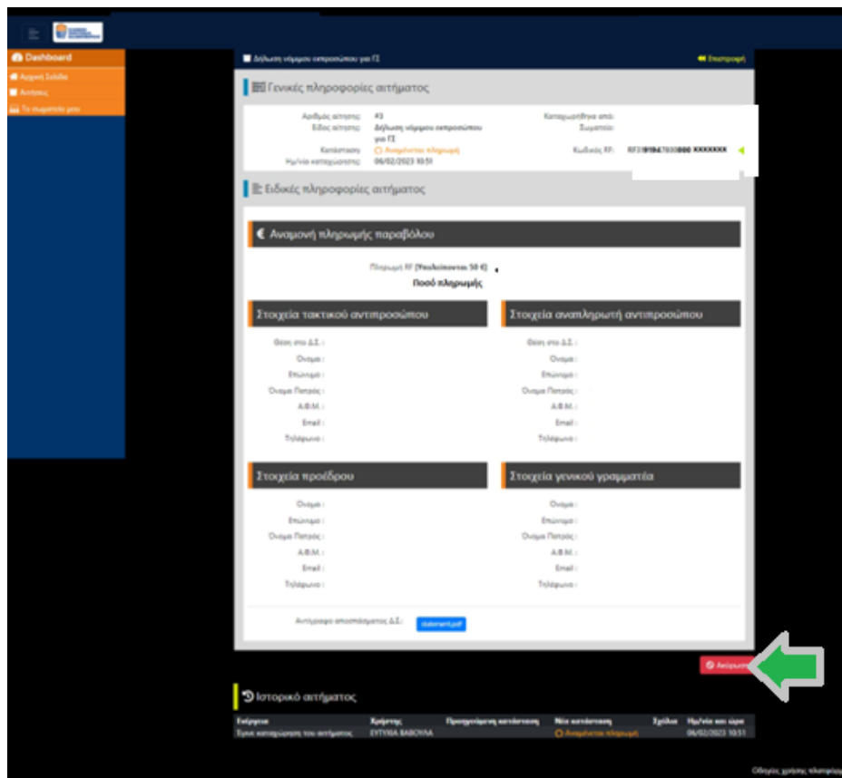
Εικόνα 12: Ακύρωση αιτήματος
